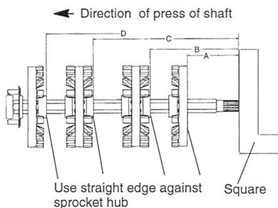
4 Drive Sprocket
