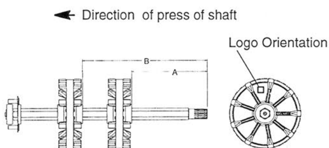
2 Drive Sprocket
